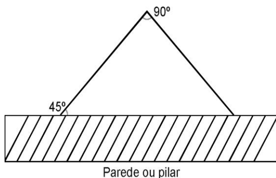
Figura 1 - Instalação de placa angular
